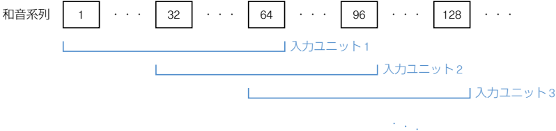
図 4 和音系列から入力ユニットへの変換 Fig. 4 Conversion from chord sequence to input unit.
